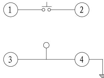
电路图
