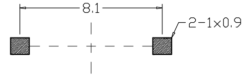
PCB线路板图
