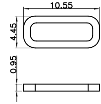
防水圈图示
