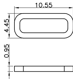
防水圈图示
