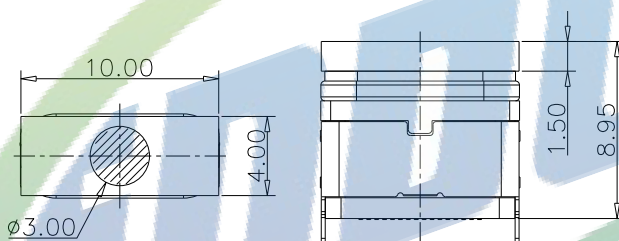
装前塞示意图
