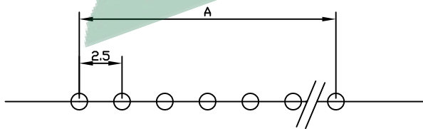
PCB寸法
